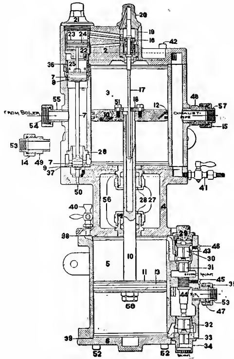
Fig. 1689. Longitudinal Section,
